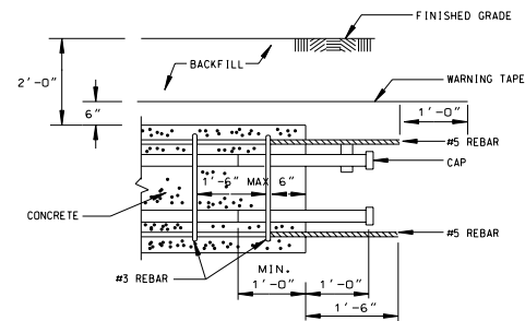
CONDUIT STUBOUT N.T.S.
