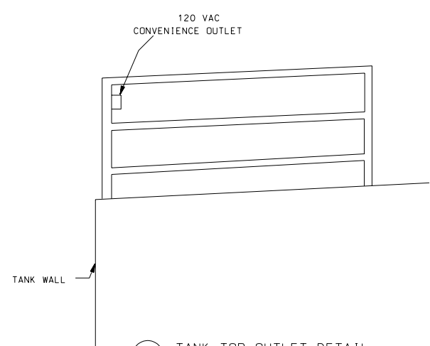
TANK TOP OUTLET DETAIL N.T.S.
