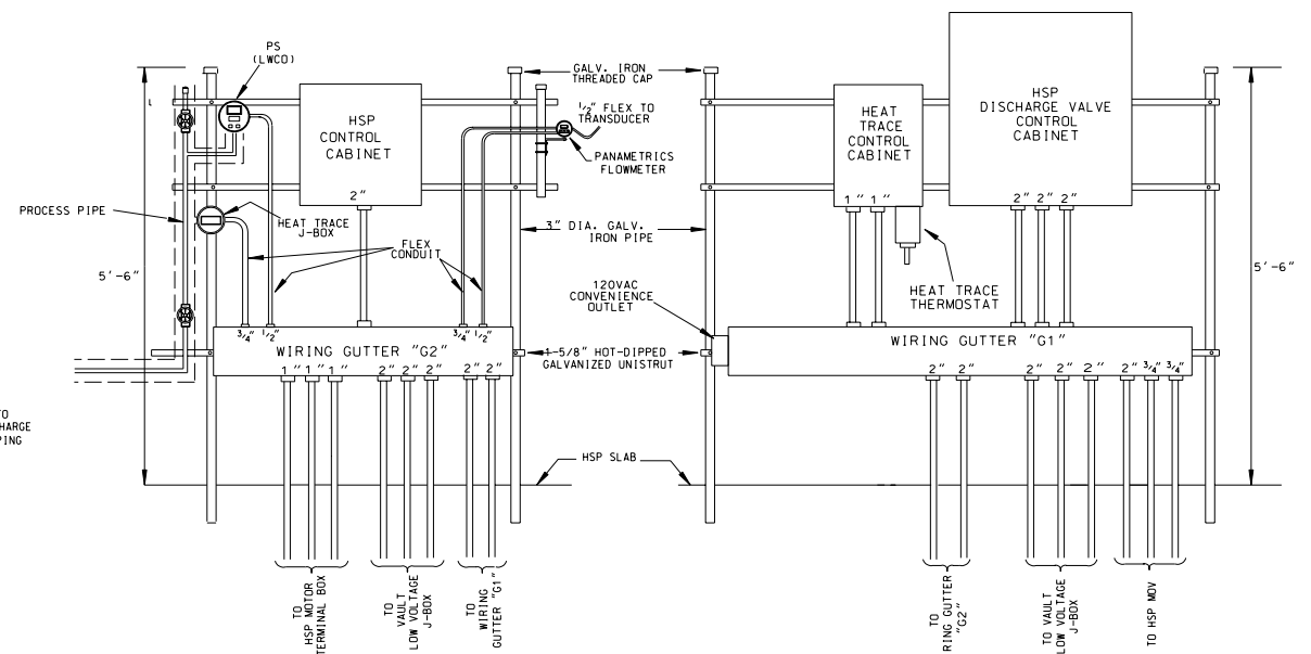
3 HSP CONTROL RACK N. T. S.
